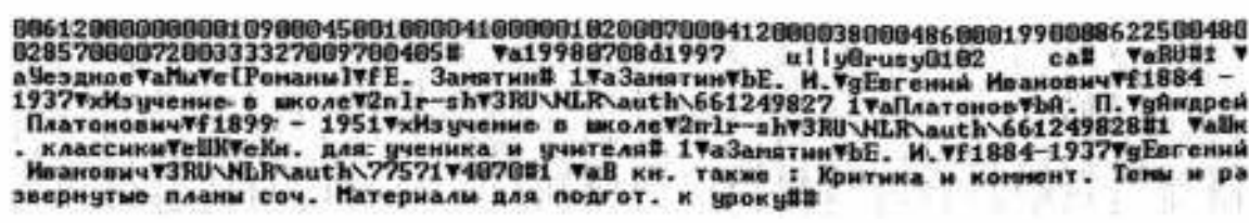
Рис. 1. Пример библиографической записи в формате ISO-2709.
