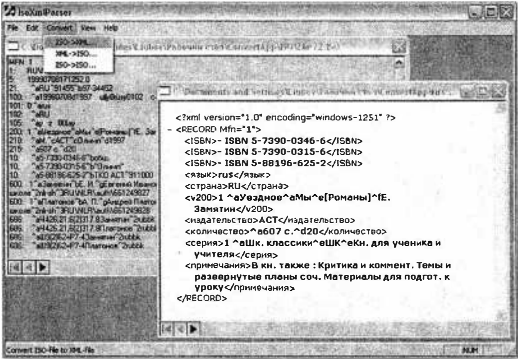
Рис. 7. Пример окон программного приложения с библиографическими записями: исходная — в формате ISO-2709, преобразованная — на языке XML.
