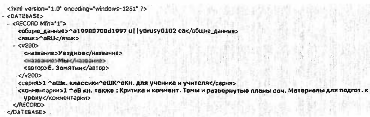
Рис. 2. Пример библиографической записи в формате XML.
