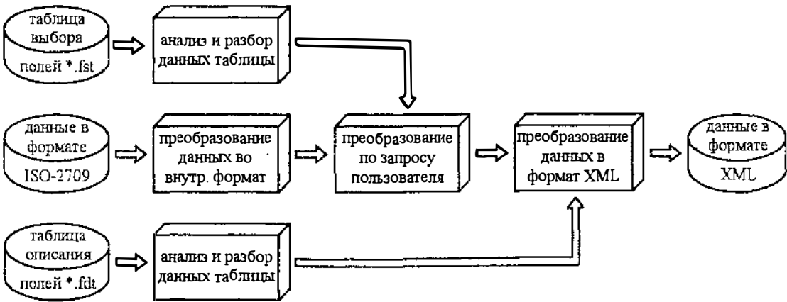
Рис. 5. Блок-схема конвертирования данных из формата ISO-2709 в формат XML.
