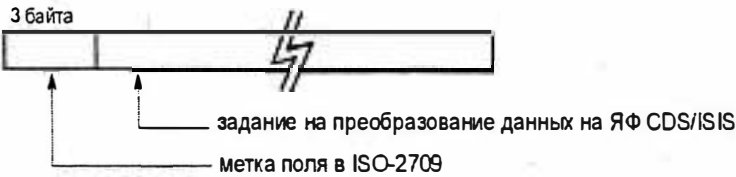
Рис. 8. Структура таблицы выбора полей.
