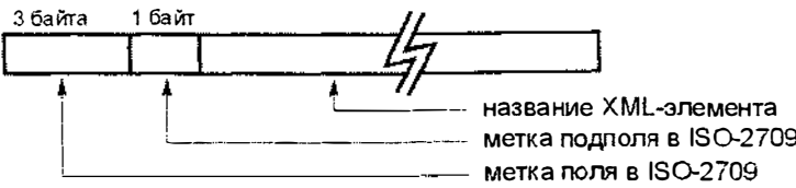
Рис. 6. Структура таблицы описания полей.
